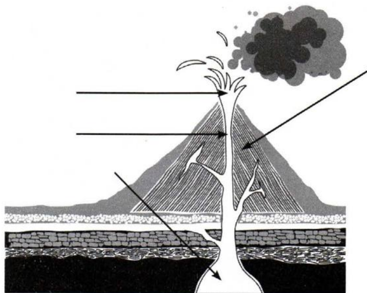
Рис. 2. Строение вулкана
